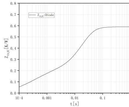
瞬态热阻抗 二极管, D5-D6 transient thermal impedance Diode, D5-D6
