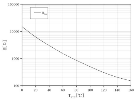
负温度系数热敏电阻温度特性 (典型) NTC-Thermister-temperature characterister(typical)
